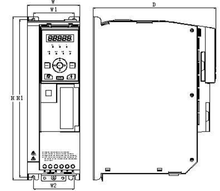
Рис. 2. IMD_E 7,5 – 15 кВт
