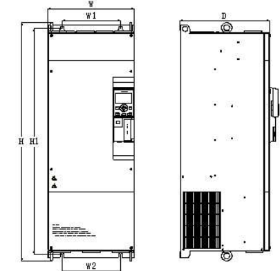
Рис. 4. IMD_E 37 – 200 кВт
