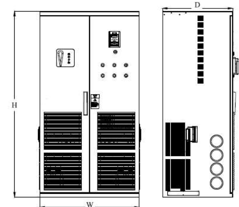
Рис. 6. IMD_E 500 – 710 кВт
